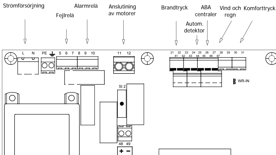
Fig. 2: Klämmornas placering
