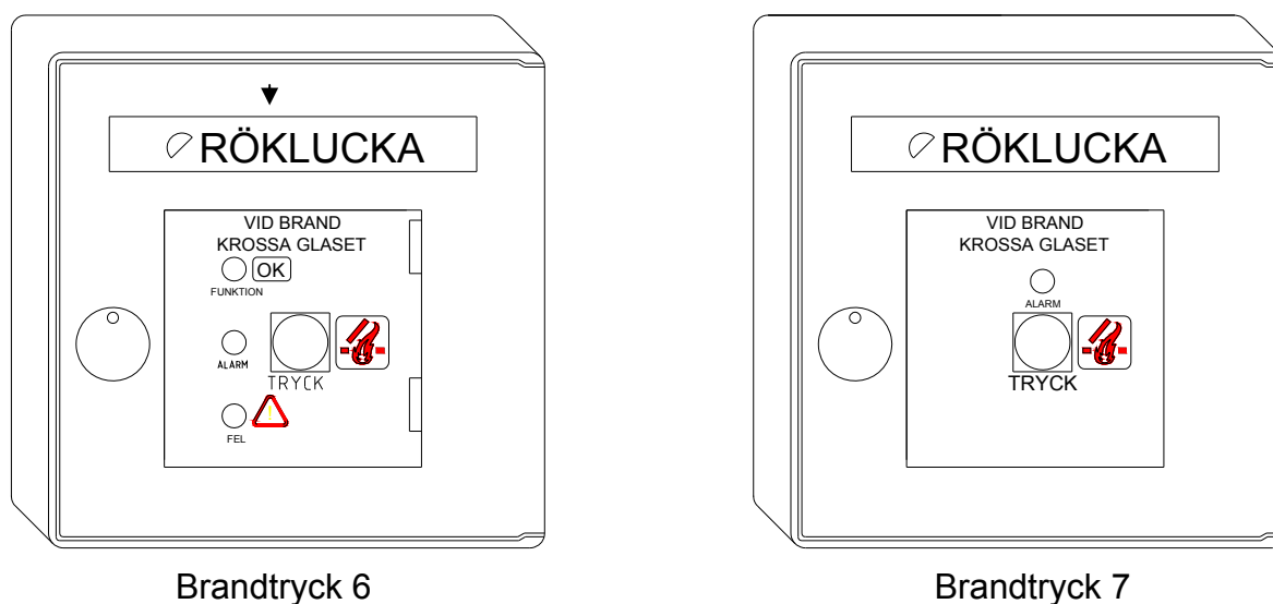
Fig. 4: Brandtryck 6 och 7
